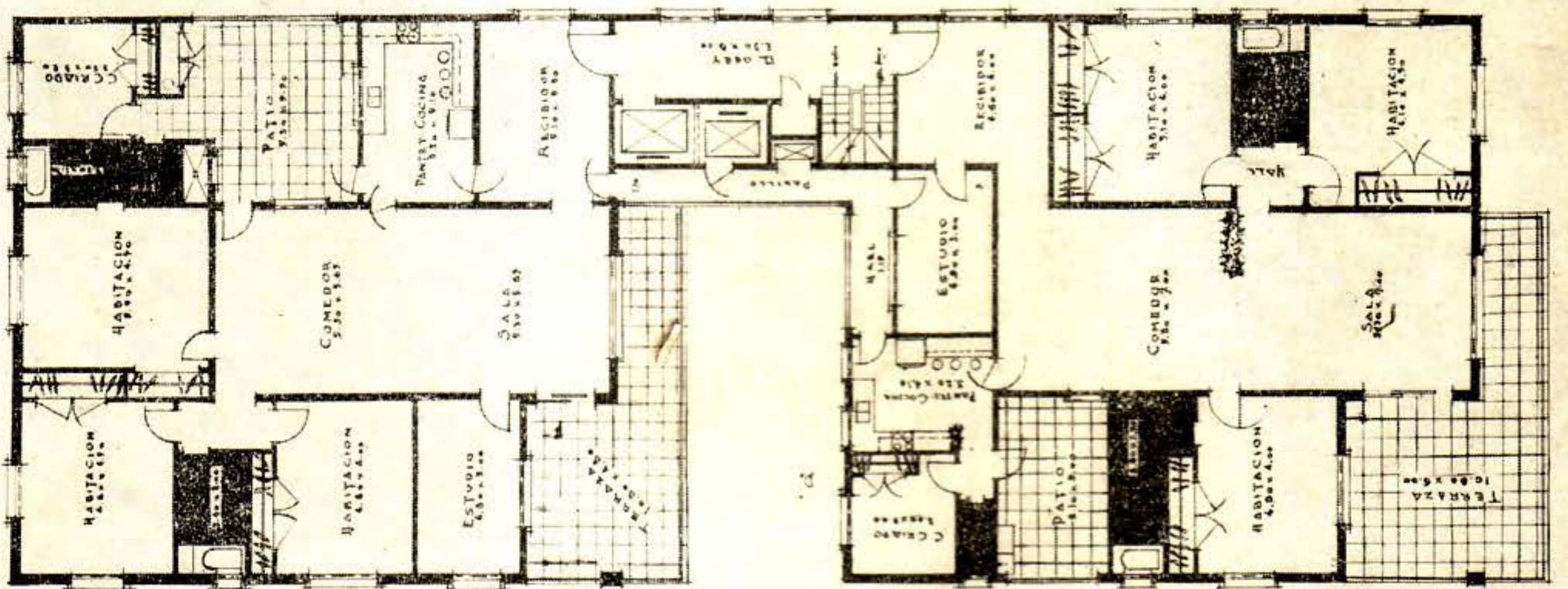
Planta típica del edificio de 15 pisos construido en el Vedado por el Arquitecto Laureano Cancio Prades, conteniendo cuatro apartamentos por piso en los cuatro bloques que forman la composición.
