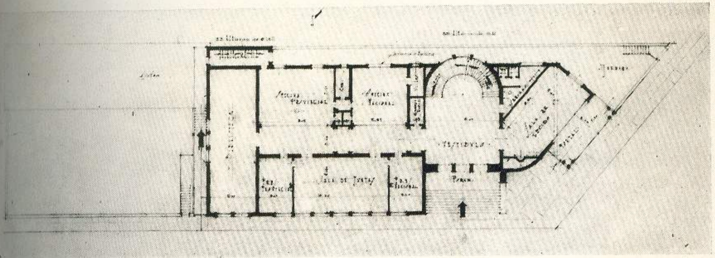
Planta baja.
