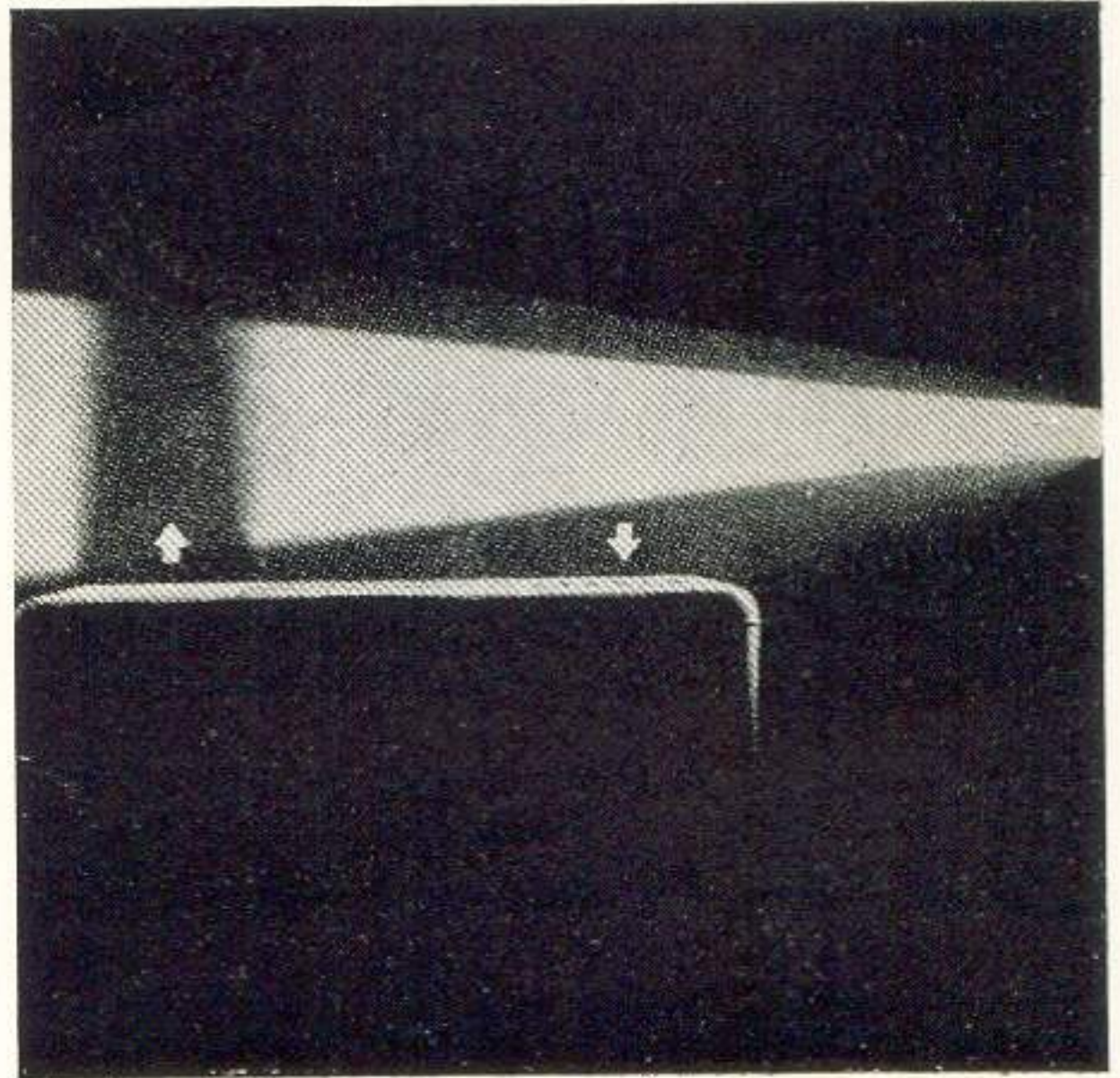
Si no fuera por el humo y el polvo no veríamos el haz de luz del proyector en los cines. La flecha de la derecha indica la entrada del aire viciado en el aparato, y la de la izquierda la salida del aire limpio de humo y polvo que forma como un corte en la cinta de luz.
