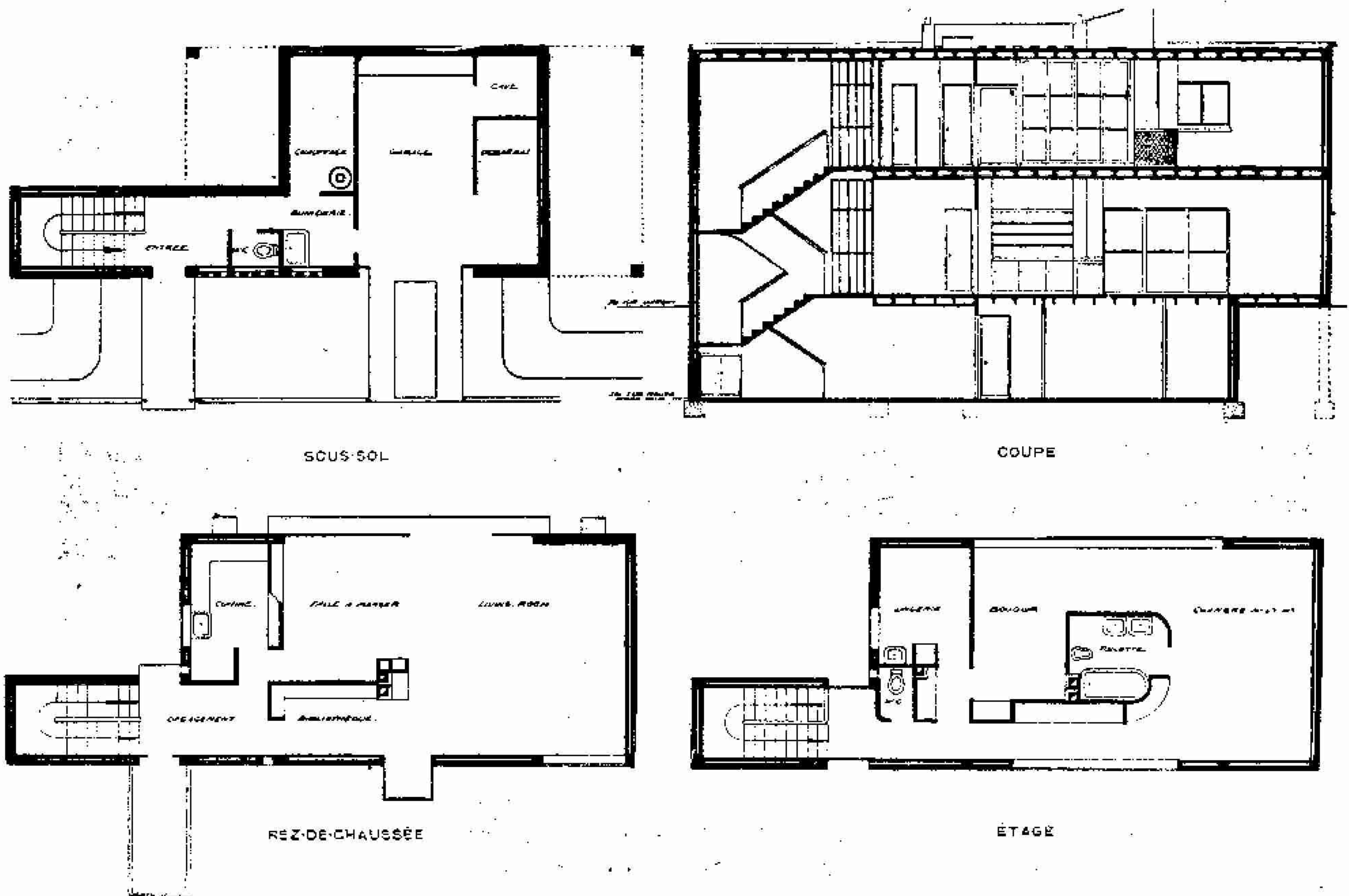
Villa a Vuoresson.--(Plantas.) Le Corbusier y P. Jeanneret, arquitectos.--1923.
