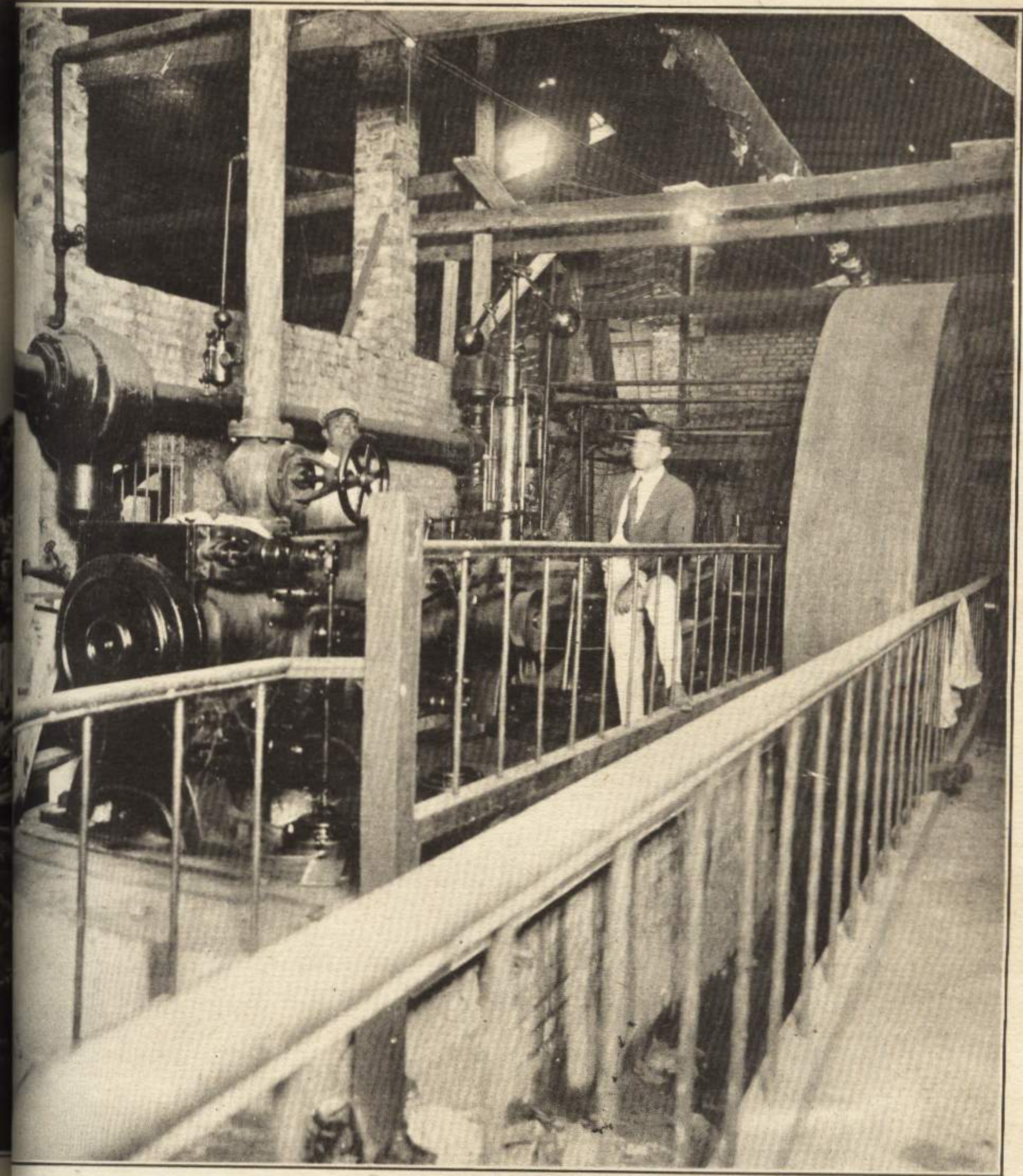
Máquinas auxiliares de vapor.
