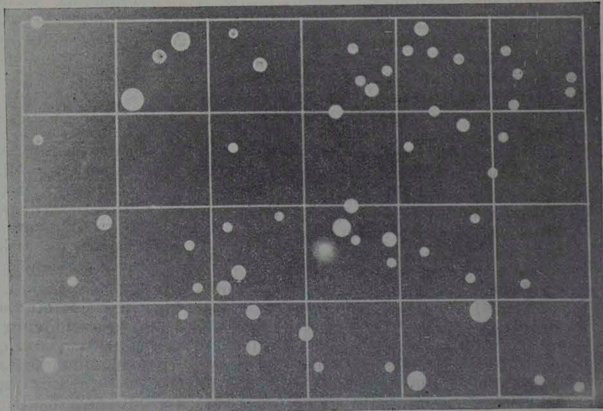
Ampliación fotográfica, del negativo del Yerkes, donde aparece, la estrella que se considera como una Nova.
