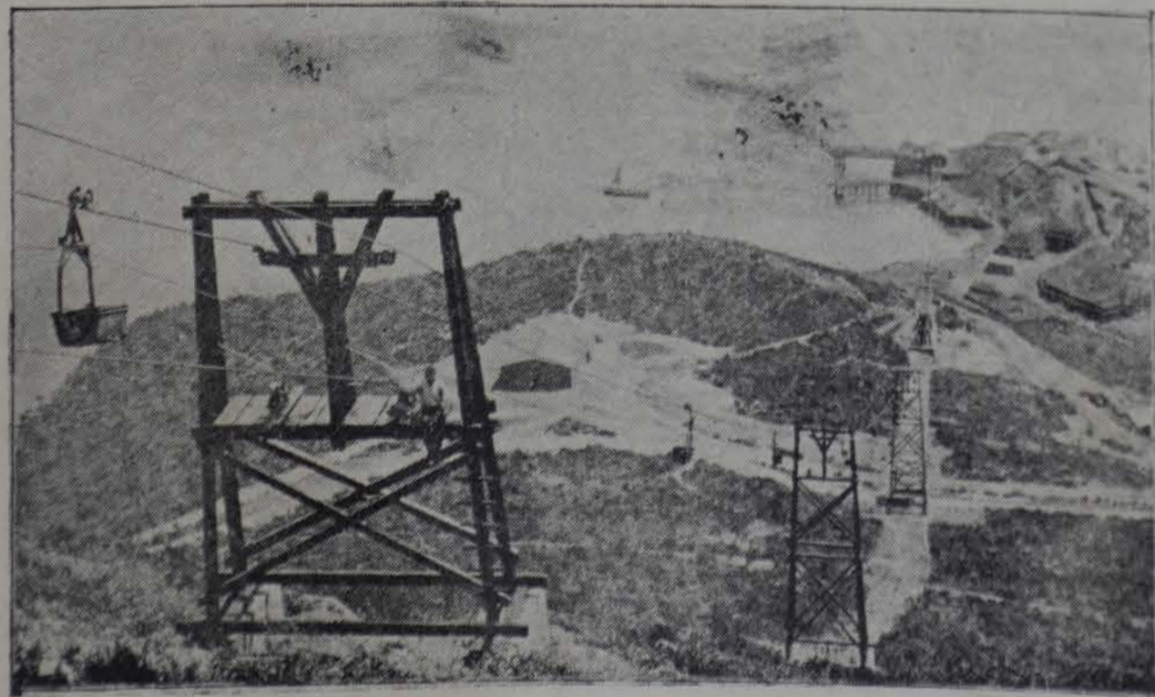
Transporte de mineral de hierro en Porto-ferrajo [Isla de Elba]
