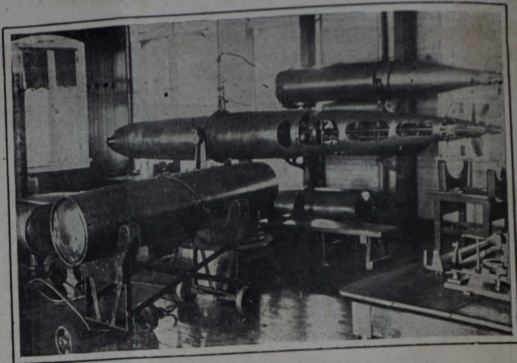
Torpedo mostrando su mecanismo interior, usado para la instrucción de los alumnos de la Escuela Naval de Torpedos
