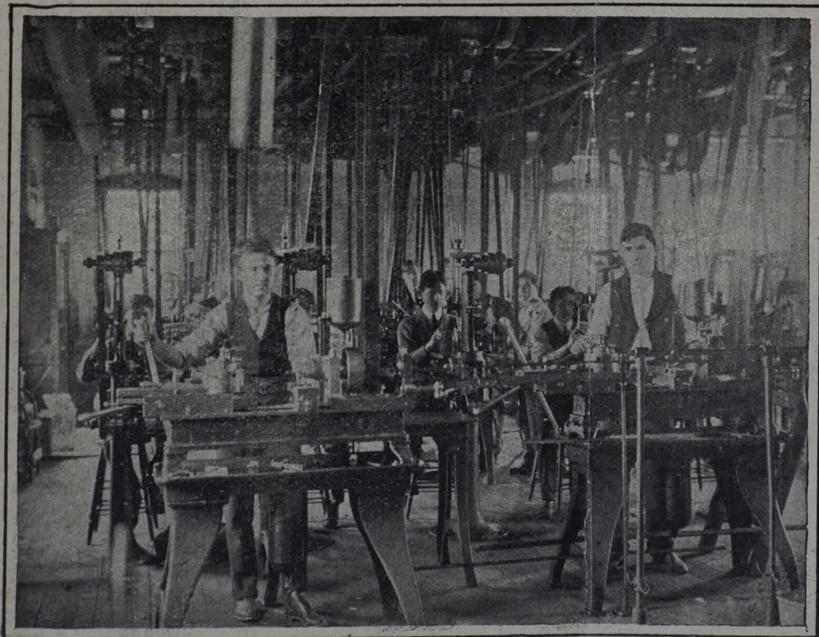
Preparando el cobre que se usa en los torpedos
