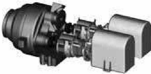
Fig. 4. Diseño del aerogenerador Bard 6,5 MW con transmisión normal doble salida.
