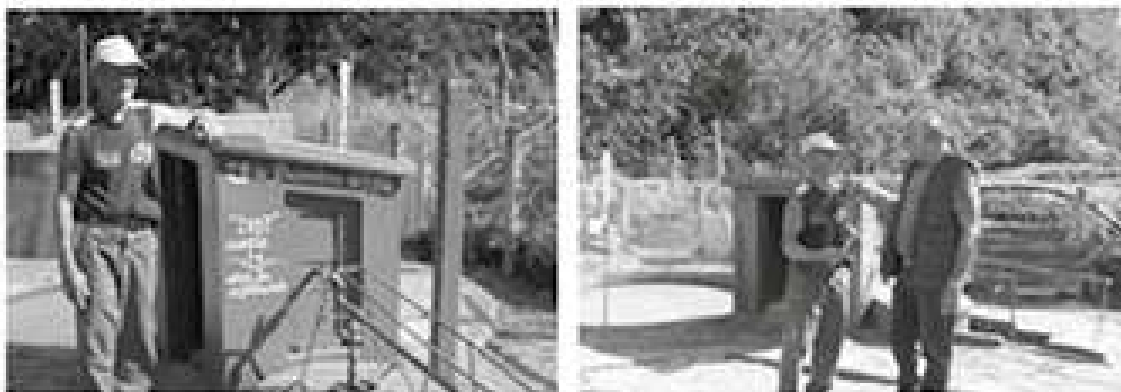
Fig. 4. Biodigestor del usuario El Papa, obra insigne en la presa Jibacoa, municipio de Manicaragua, Villa Clara.
