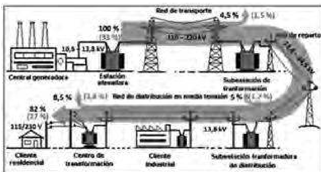
Fig. 2. Pérdidas en la red eléctrica.
