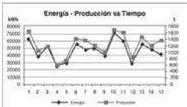
Fig. 1. Gráficos de control de energía–producción contra tiempo.
