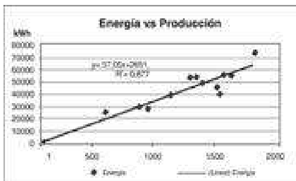
Fig. 2. Gráficos de control de energía contra producción.
