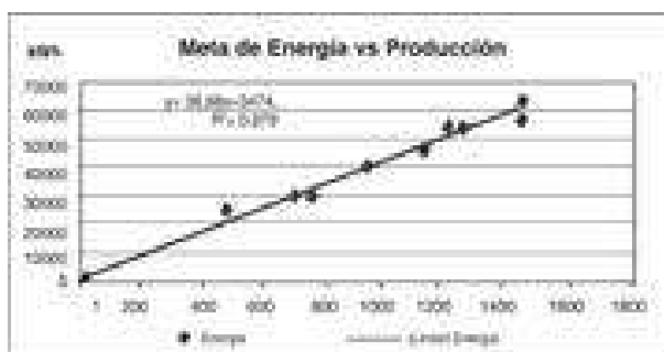
Fig. 3. Meta de energía contra producción.
