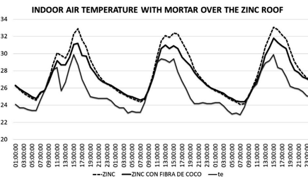
Fig. 8. Temperatura del are interior en el módulo experimental añadiendo mortero con fibra de coco sobre el techo de «zinc». Mediciones realizadas en un día nublado y un día lluvioso de abril, 2016.
