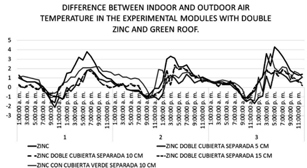
Fig. 9. Diferencia de la temperatura de aire interior con respecto al exterior en el módulo experimental con doble cubierta. Mediciones realizadas en marzo de 2016. Primera noche lluviosa y segundo día lluvioso para la cubierta verde doble
