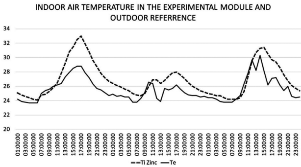
Fig. 6. Temperatura del aire interior en el módulo experimental con techo de «zinc».
