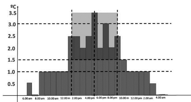
Fig. 12. Combinación de histogramas que representan la distribución de valores de la diferencia entre la temperatura interior con respecto al exterior, medido en las viviendas y en los módulos experimentales con techo sencillo de «zinc».
