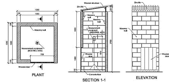
Fig. 2. Módulo experimental.
