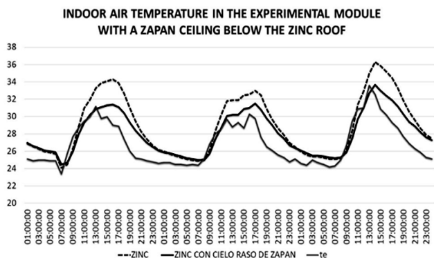
Fig. 11. Temperatura del aire interior en el módulo experimental adicionando un falso techo de «zapán» a la cubierta de «zinc». Mediciones realizadas en días soleados y la última noche lluviosa, marzo 2016.
