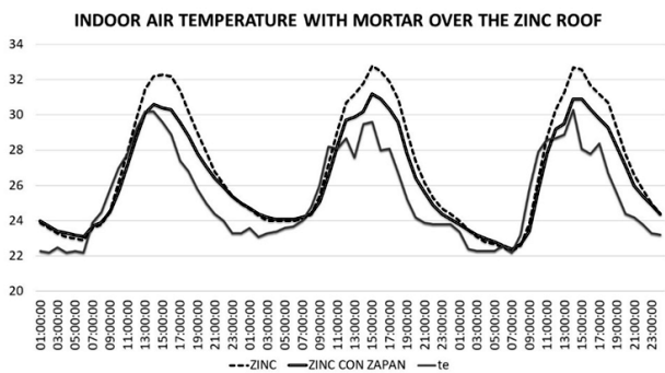
Fig. 7. Temperatura del aire interior en el módulo experimental adicionando mortero con «zapán» sobre el techo de «zinc». Mediciones realizadas en un día soleado de abril, 2016.
