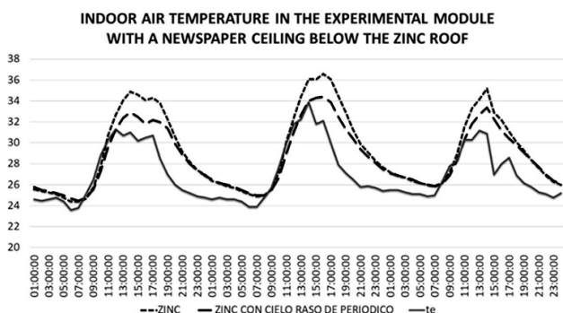
Fig. 10. Temperatura del aire interior en los módulos experimentales adicionando un falso techo de periódico a la cubierta de «zinc». Mediciones realizadas en días soleados y la última tarde lluviosa, marzo de 2016.
