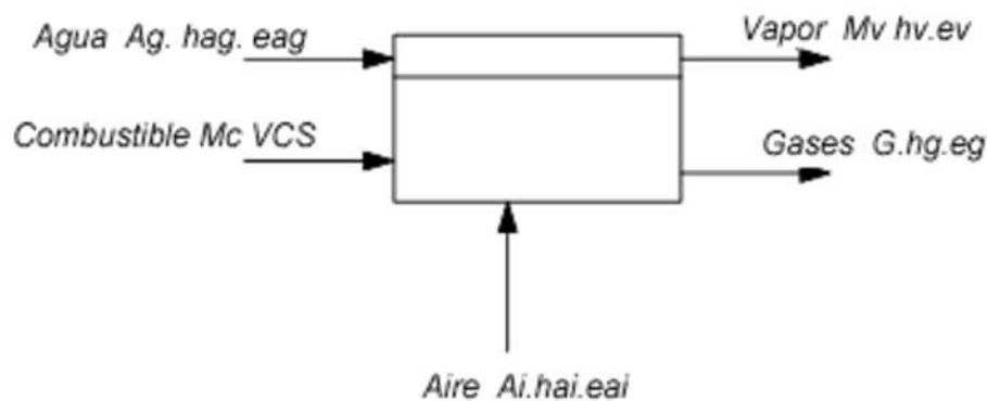
Fig. 2. Esquema del proceso de generación de vapor
