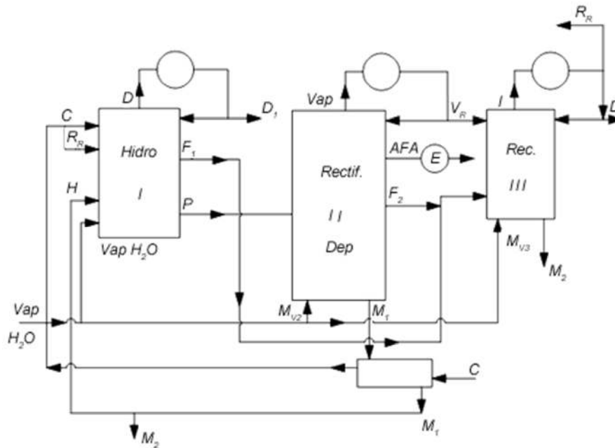
Fig. 1. Esquema de distribución y uso del vapor en la destilería
