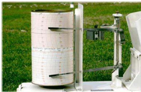
Fig. 1. Higrotermógrafo. Registra en una gráfica de papel, simultáneamente, la temperatura (en °C) y la humedad relativas del aire (en %).
