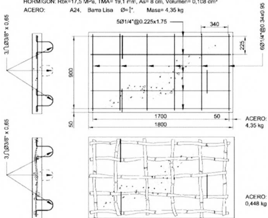
Armadura de la losa ET 84-02
