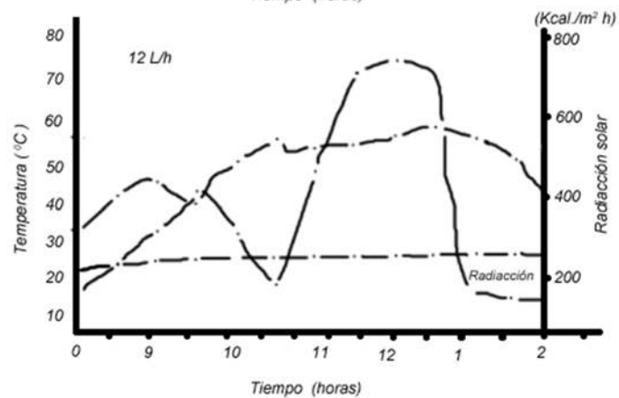
Figs. 2 y 3. Curvas de temperatura de entrada y salida de un colector solar plano a flujos de 6 y 12 L/h, y curvas de radiación solar correspondientes a los días en que se realizó la prueba
