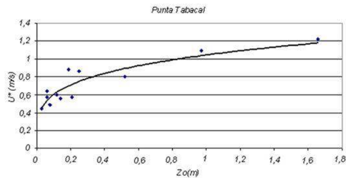
Fig. 18. Relación Z_0 vs. u^* para la estación de Punta Tabacal.
