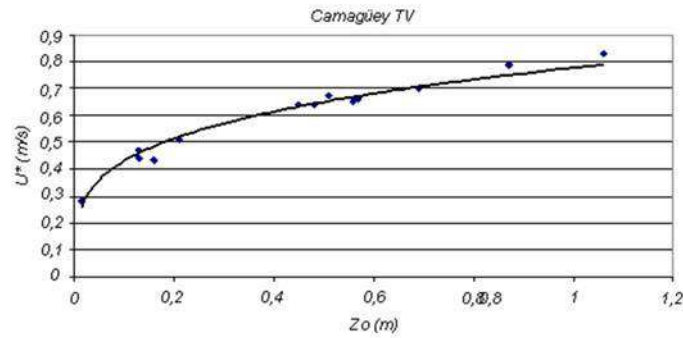
Fig. 17. Relación Z_0 vs. u^* para la estación de Camagüey.
