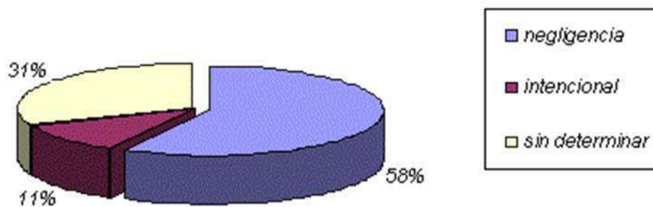
Anexo 3. Causas que provocaron los incendios forestales
