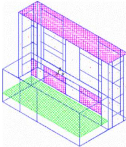
Fig. 5. Modelo geométrico elaborado en ADELINÉ del edificio ubicado en Reina 412, entre Gervasio y Escobar, Centro Habana. (Tomado de Gómez, 2005).
