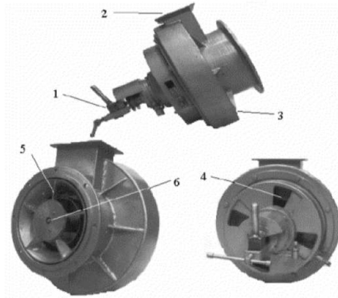
Fig. 6. Quemador rotatorio combinado de 1 MW, diseñado para quemar combustible líquido y residuos biomásicos pulverizados (Patente: 22526). 1. Caña del combustible líquido. 2. Conducto de entrada del combustible sólido. 3. Cuerpo del ventilador. 4. Válvula del aire. 5. Estabilizador rotatorio de dos corrientes. 6. Boquilla del combustible.
