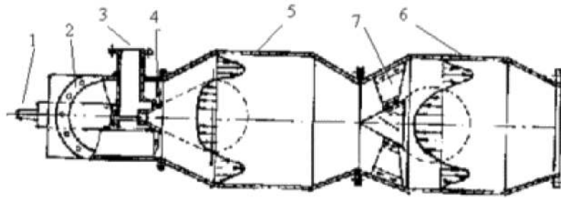
Fig. 2. Secador dinámico. 1. Sistema matriz. 2. Entrada de gases. 3. Conducto de alimentación del bagazo húmedo. 4. Impelente estabilizador. 5. Segundo cuerpo. 6. Tercer cuerpo. 7. Estabilizador estático.
