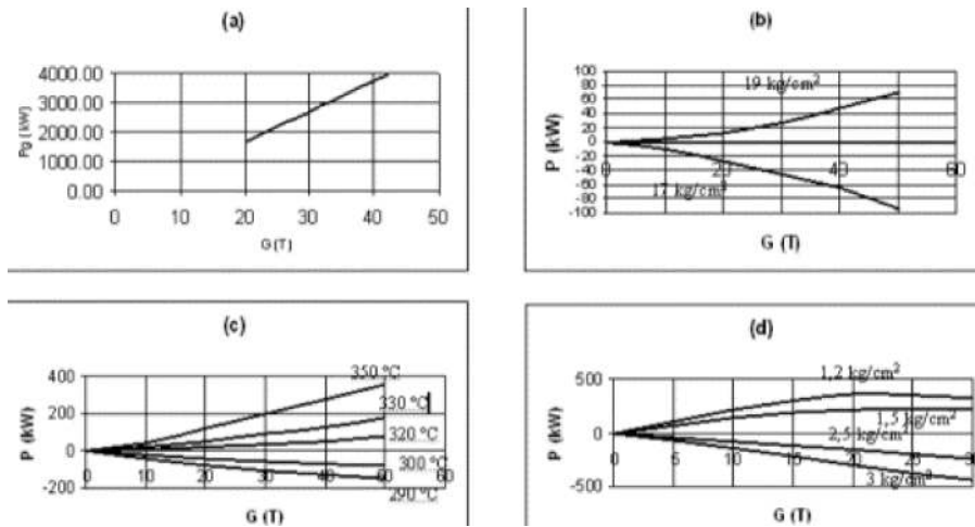
Fig. 1. Características de explotación del turbogenerador. a) Dependencia de la potencia eléctrica respecto al consumo de vapor para P_0 = 18 \text{ kg/cm}^2 \text{ abs} , T_0 = 310 \text{ °C} y P_2 = 2 \text{ kg/cm}^2 \text{ abs} . b) Corrección por presión de vapor directo. c) Corrección por temperatura del vapor directo. d) Corrección por presión de escape.
