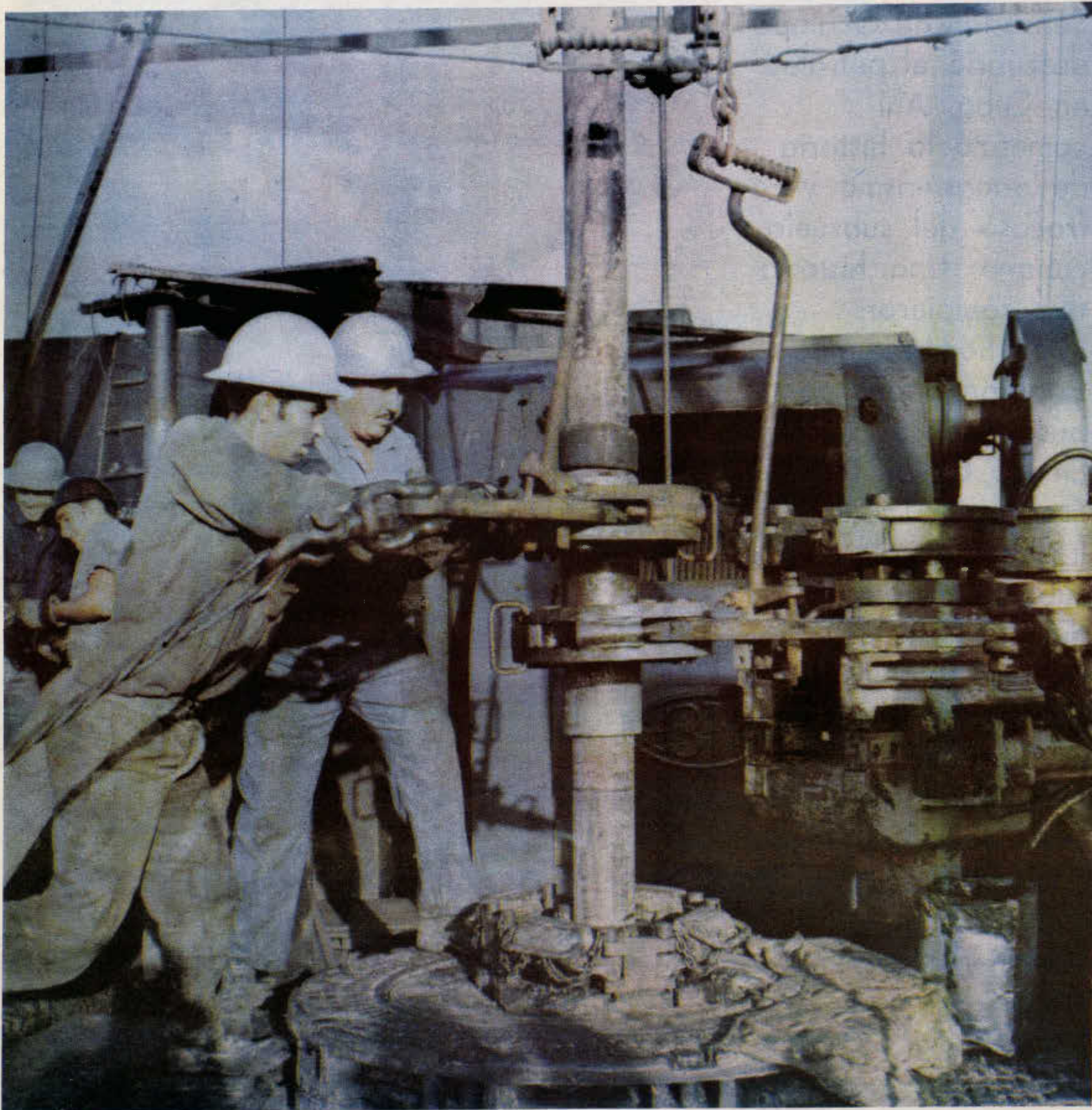
INTRODUCIENDO LA BARRENA EN EL POZO
