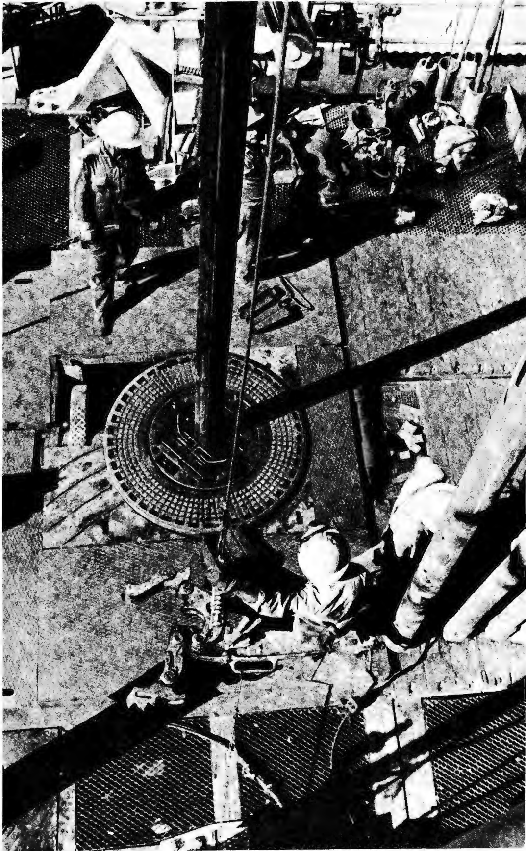
LAS BARRAS PERFORADORAS ENTRAN EN LA MESA DE ROTACION
