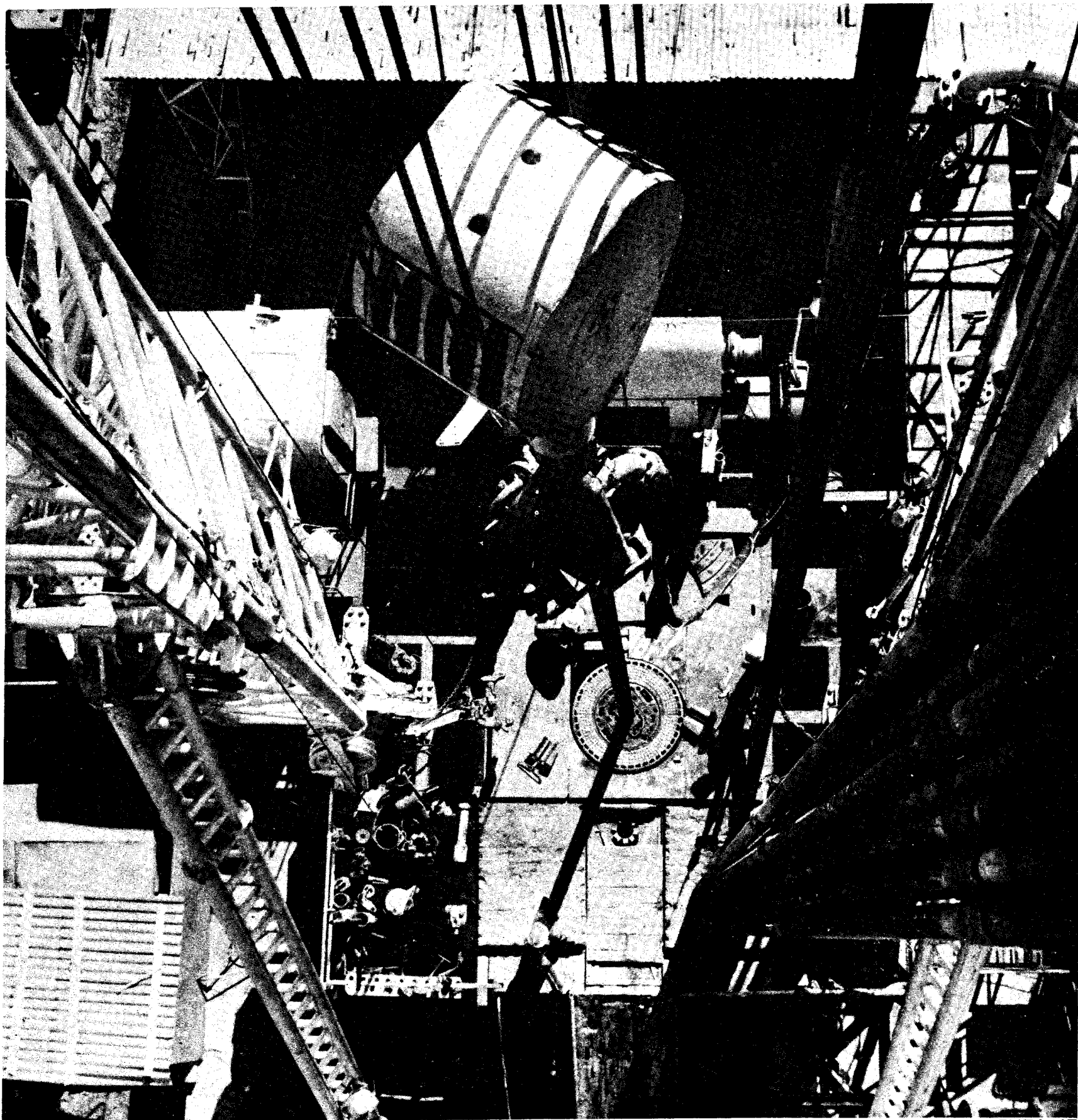
ASI VE EL TORRERO LOS TRABAJOS DEL APAREJO Y LA MESA DE ROTACION. EN LA FOTO LA TORRE RUMANA: 41 METROS DE ALTURA
