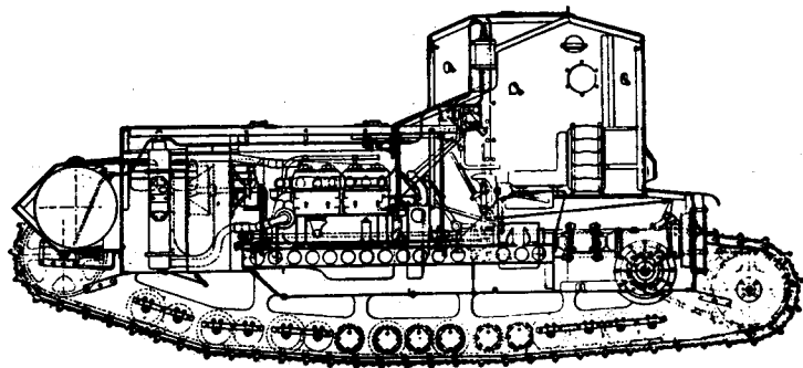
CORTE VERTICAL DEL TANQUE MARK A
