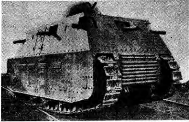
EL ANTIGUO TANQUE PESADO "FIAT"
