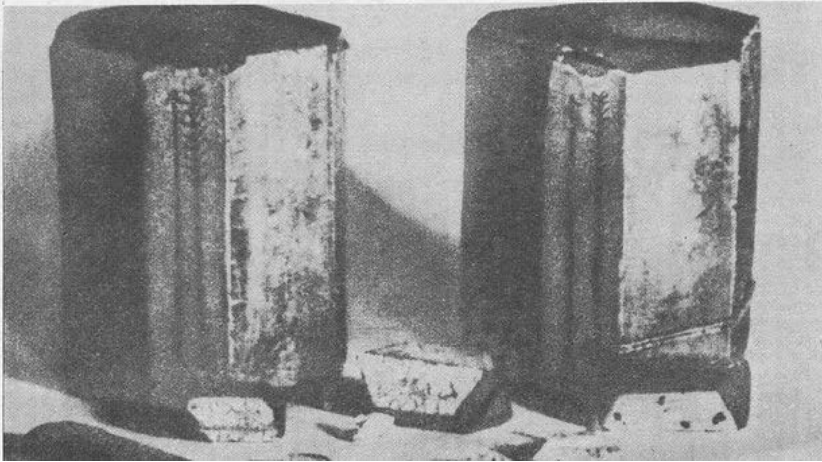
En 1847, Pasteur se graduó en Química. El año siguiente —tenía sólo 26 años— terminó sus estudios sobre la asimetría de los cristales de las sales del ácido tartárico y atribuyó a las moléculas de dicho ácido la causa de tal asimetría. Debajo: modelos de cristales de tartrato sódico hechos por Pasteur en corcho. Arriba a la derecha: Pasteur en 1849 siendo profesor de Strasburgo. A la izquierda: María Laurent, hija del Decano de la Universidad de Strasburgo, que se casó con Pasteur el 21 de Mayo de 1849.
