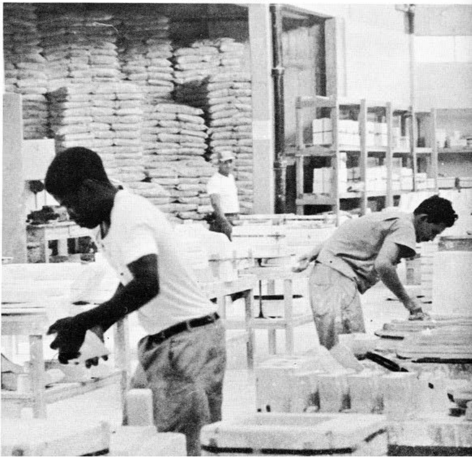
UN ASPECTO DE LA SECCION DE MOLDES Y MATRICES. AQUI TRABAJAN NUEVE OBREROS ESPECIALIZADOS QUE PRODUCEN UNOS 10 MOLDES DIARIOS. DE CADA UNO DE ESTOS MOLDES PUEDEN SALIR HASTA CIEN PIEZAS.
