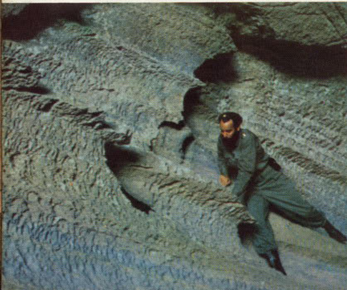
LA EROSION DE LOS RIOS SUBTERRANEOS ORIGINA CURIOSAS FORMAS EN LAS ENTRANAS DEL SUBSUELO: AQUI SE DESTACAN LAS TRINCHERAS INCLINADAS DE LAS MARGENES DEL RESOLLADERO DEL CUYAGUATEJE.
