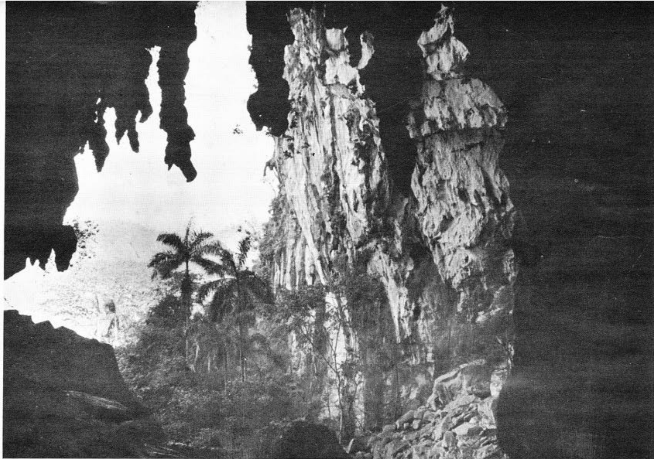
ENTRADA DE LA CAVERNA DEL SUMIDERO POR DONDE PENETRAN LAS AGUAS DEL RIO CUYAGUATEJE.
