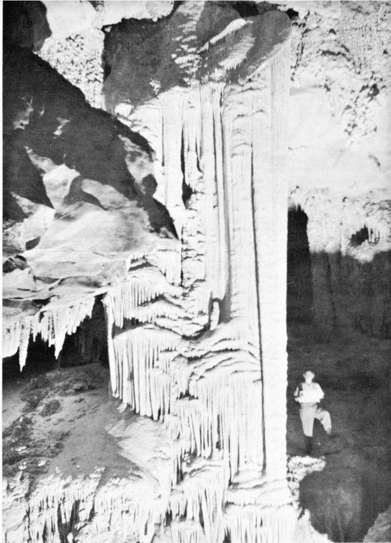
COLUMNA DE LA CUEVA DE LAS ANTORCHAS, EN EL SISTEMA SUBTERRANEO DE LA "GRAN CAVERNA DE SANTO TOMAS", EN PINAR DEL RIO.
