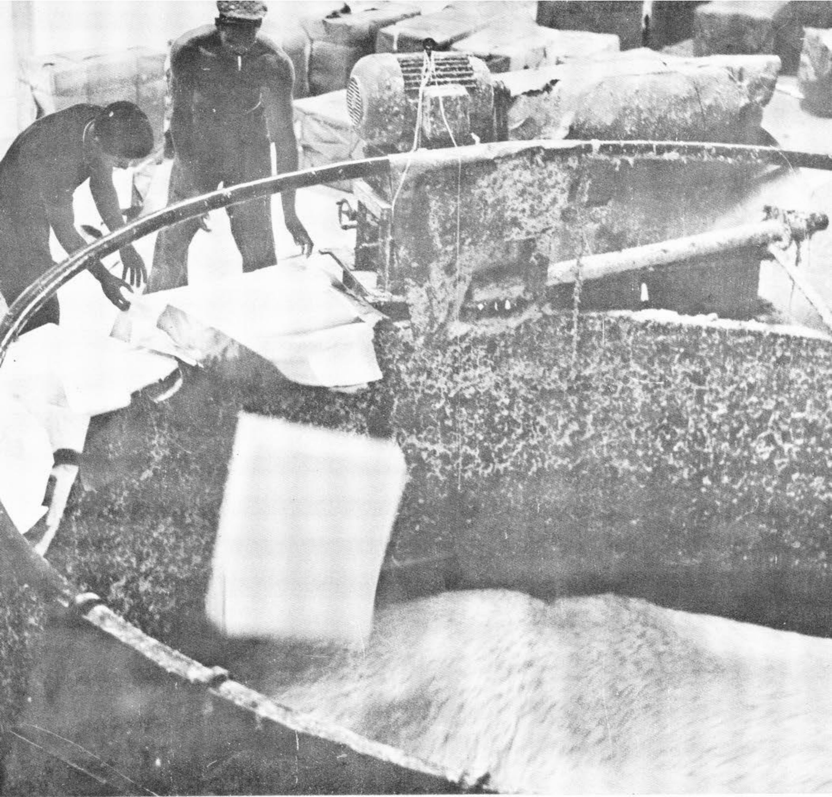
Dos obreros adicionan la pulpa al bagazo que se encuentra en los tanques. Ahora se industrializa lo que antes se quemaba en las calderas.
